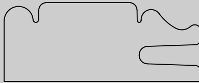
Miter 33 DF
